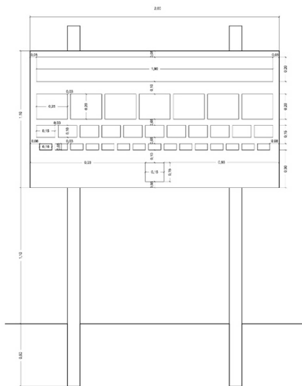
Modelo 1.1: Placa Identificativa única dos colaboradores/doadores de Bens e Serviços Desenho técnico cotado em escala 1:15 e desenho humanizado, folha 01 de 05
